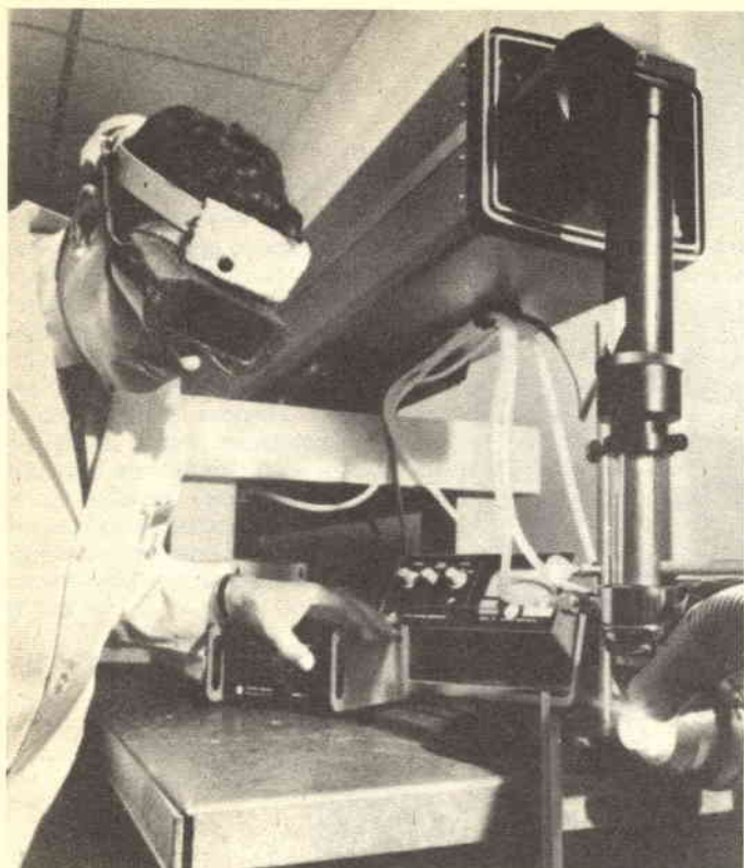
Un tubo di quarzo viene tagliato con un laser al biossido di carbonio prodotto dalla Sylvania.
