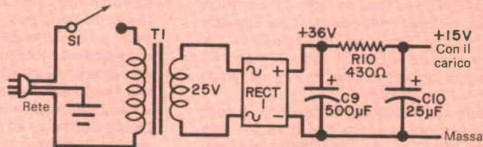
Fig. 2 - Ecco l'alimentatore da usare se i 15 V a 85 mA non possono esser ottenuti diversamente.
