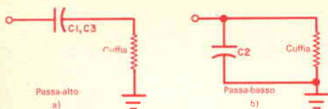
Fig. 2 - Il filtro passa-alto (a) attenua le frequenze basse; il filtro passa-basso (b) scarica a massa le frequenze alte.
