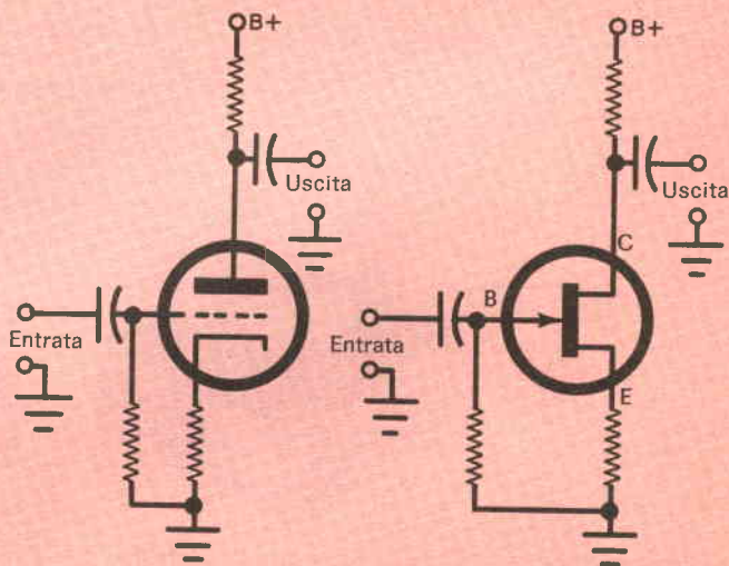
Fig. 3 - I sistemi di polarizzazione del transistoro JFET di tipo n e del triodo a vuoto sono uguali.
