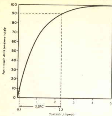
Fig. 3 - Questa è la curva della costante di tempo per la carica di un condensatore in un circuito RC in serie.
