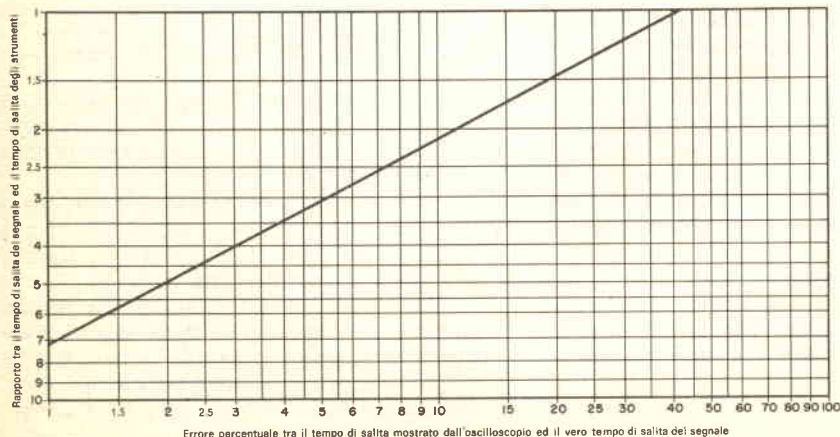
Errore percentuale tra il tempo di salita mostrato dall'oscilloscopio ed il vero tempo di salita del segnale
