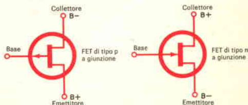
Fig. 2 - Ecco i simboli schematici per i transistori ad effetto di campo con giunzione di tipo p (a sinistra) e di tipo n (a destra).
